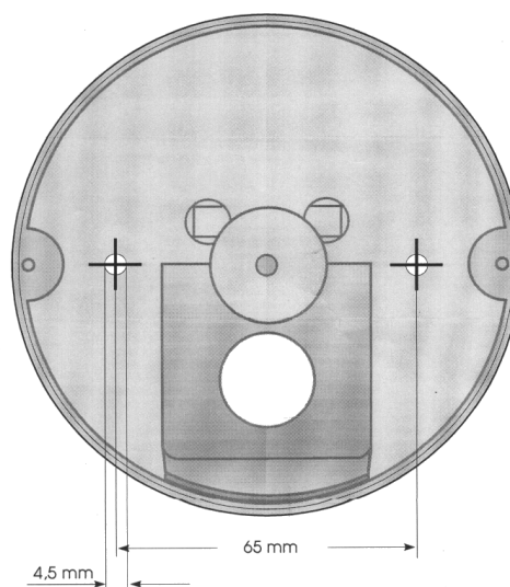
Befestigungsbohrungen im Unterteil
