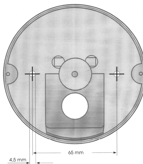
Befestigungsbohrungen im Unterteil
